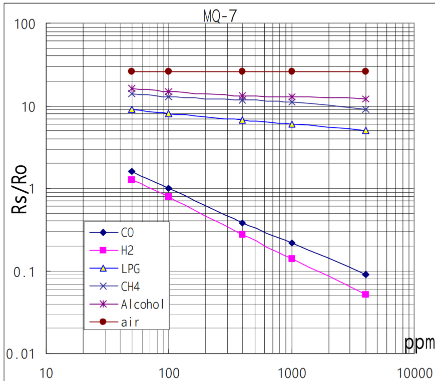
Die Abbildung zeigt die typische Empfindlichkeitscharakteristik des MQ-7. R_s bedeutet Widerstand des Sensors bei verschiedenen Gasen, R_o bedeutet
