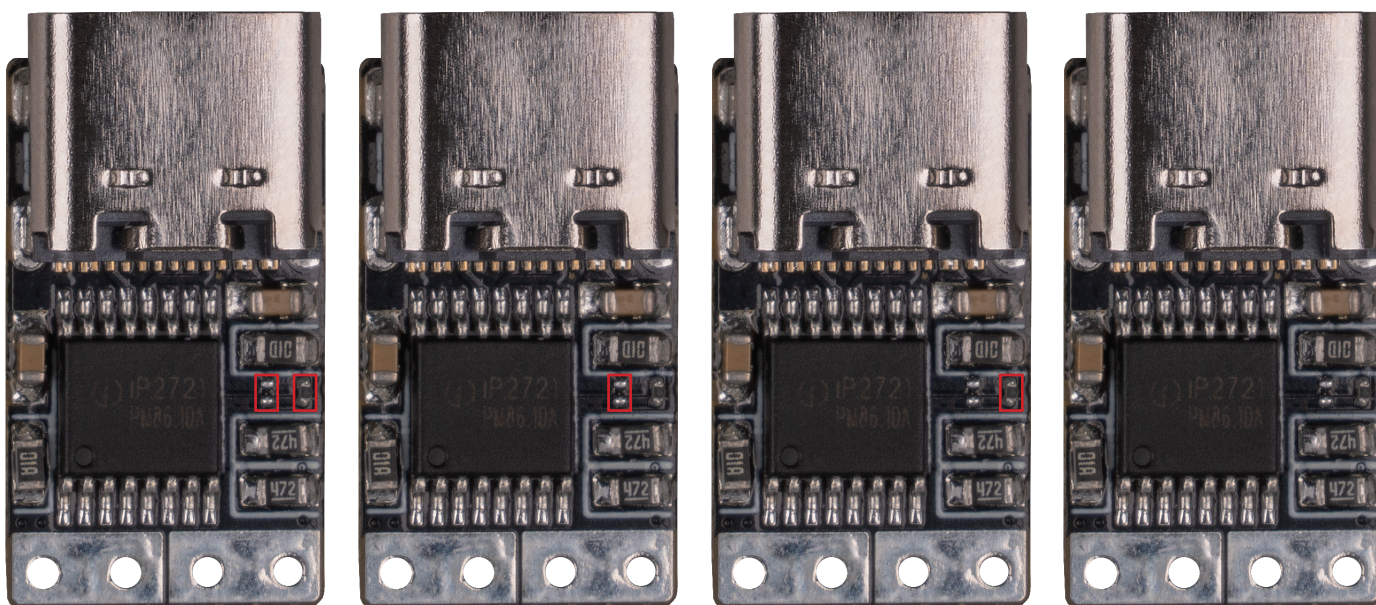
Beide Widerstände eingelötet = 5 V
