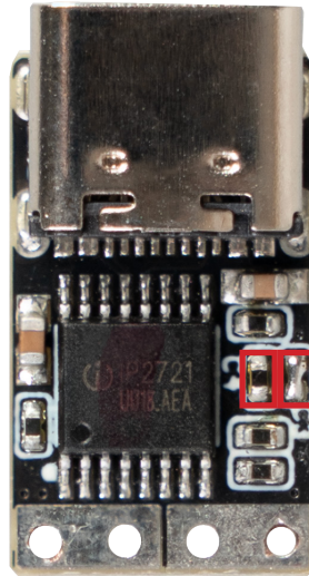
C3 & C4 entfernt = 9 V
